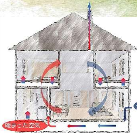
パッシブ換気の空気の流れ
